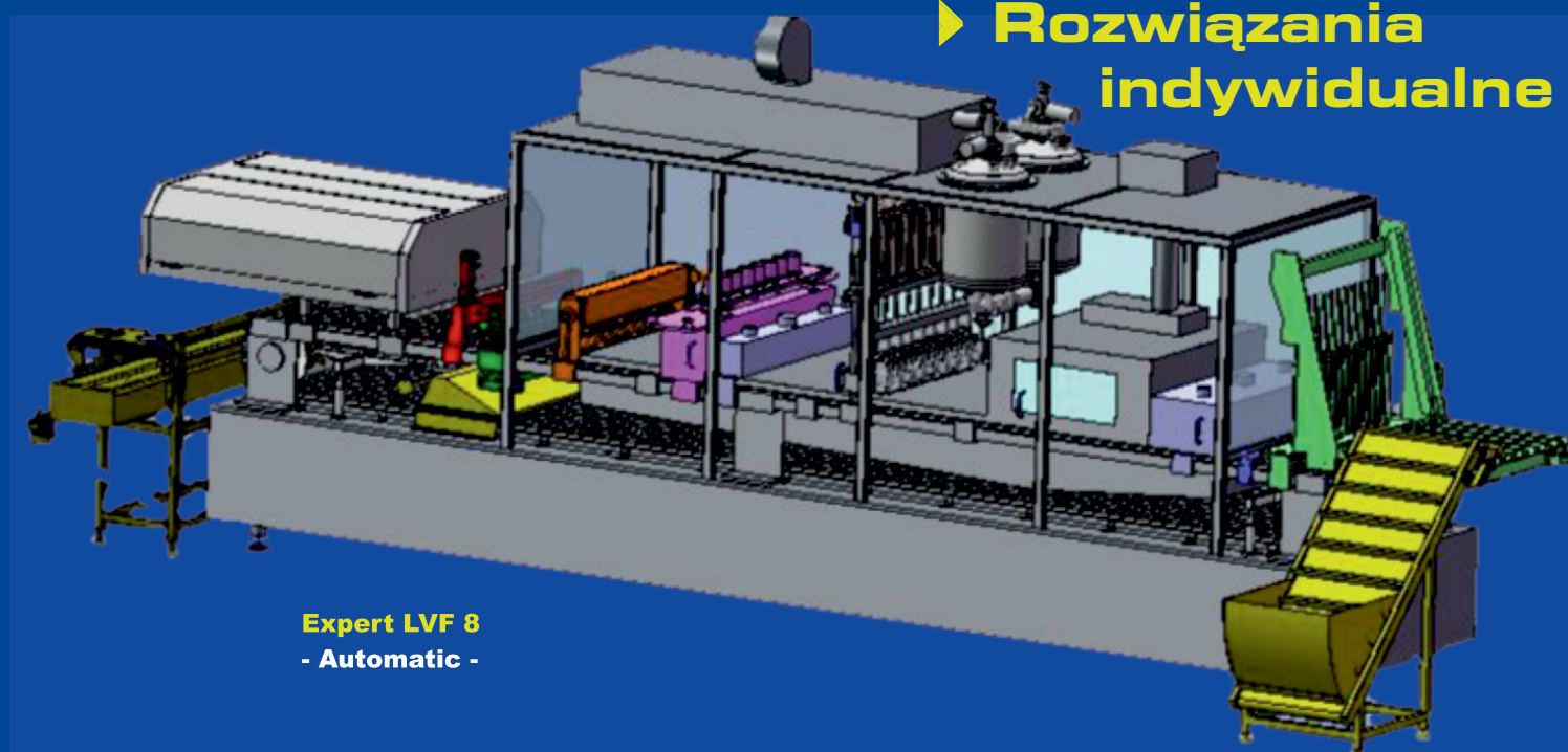
specjalny, buforowy zasobnik wieczek, wysuwany poza strefę roboczą dla wyższej higieny i łatwości obsługi special lids buffer magazine pulled out of the working zone for easy operation and improved hygiene
